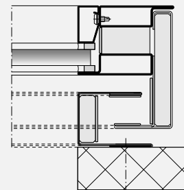
Neues Labyrinthprofil
