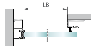
1-flügelig ohne Seitenteil Wandmontage
