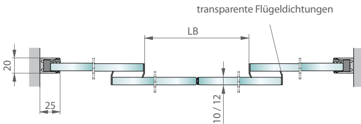
2-flügelig mit Seitenteil Wandmontage
