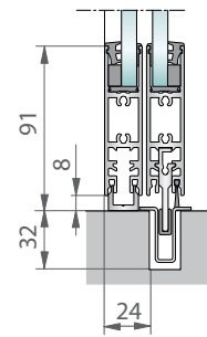
durchgehende Bodenführung mit Schuhprofil
