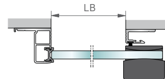
Sturzmontage
