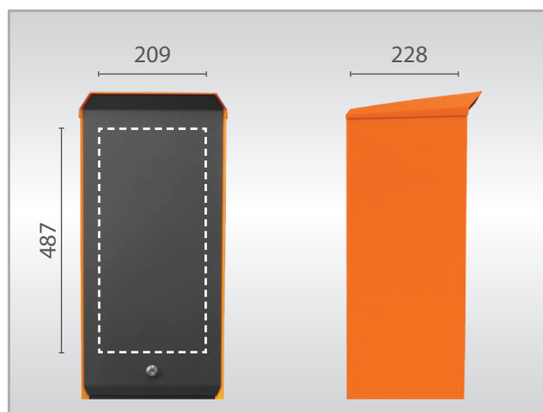
Einbaumaße Terminal MH (in mm)
