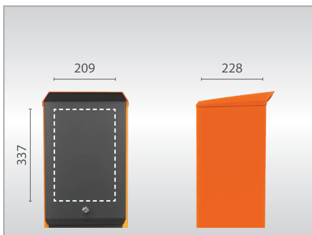
Einbaumaße Terminal MS und ML (in mm)
